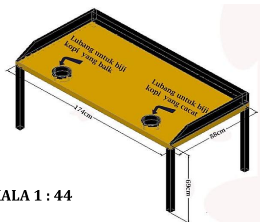
Gambar 2. Rancangan Meja Sortir Kopi beserta Ukurannya
