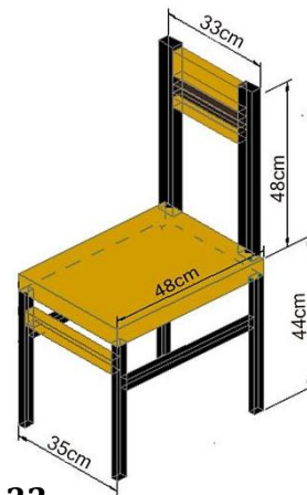
Gambar 3. Rancangan Kursi Kerja beserta Ukurannya
